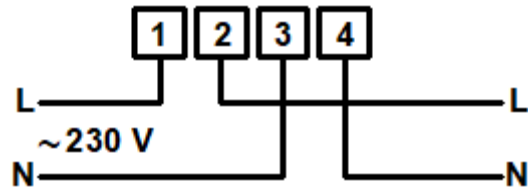
Рисунок А-1. Схема подключения счетчика в корпусе С01
